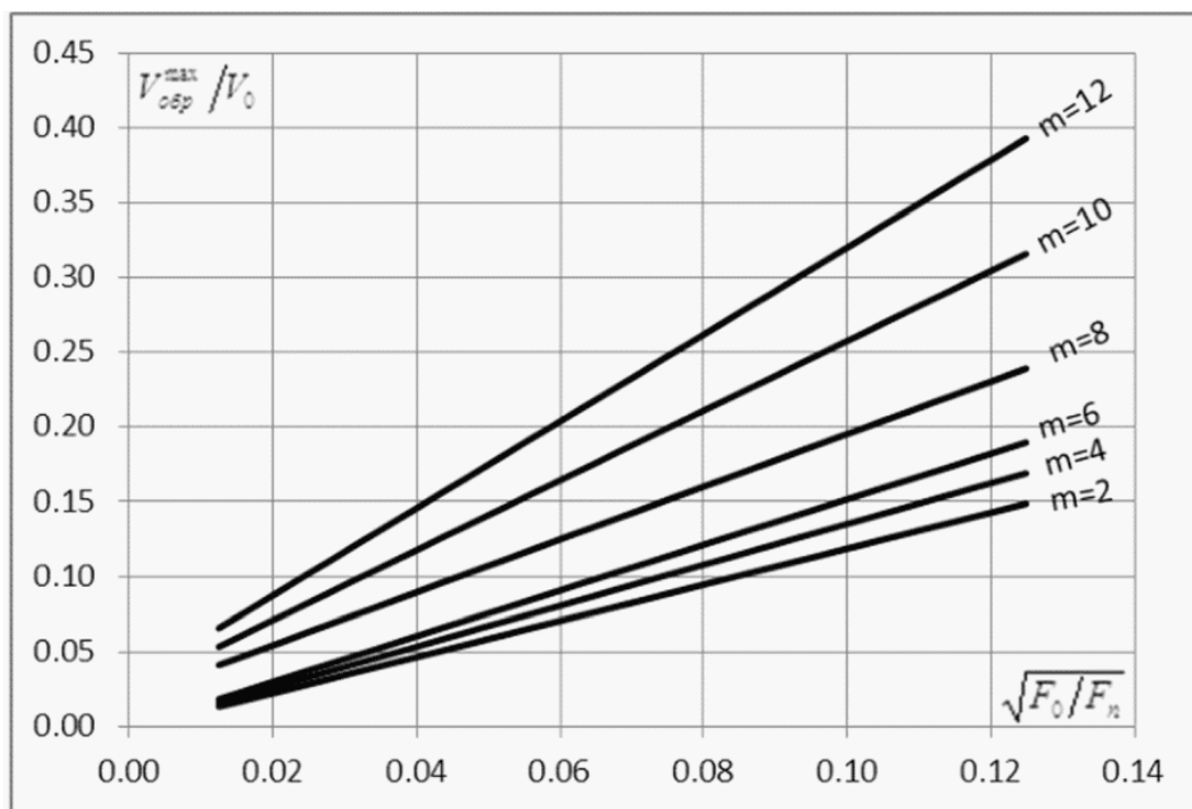
Рисунок Ж.2 - Зависимость максимальной скорости в обратном потоке от параметра \sqrt{F_0 / F_{\text{II}}} стеснения и кинематического коэффициента m ВР
