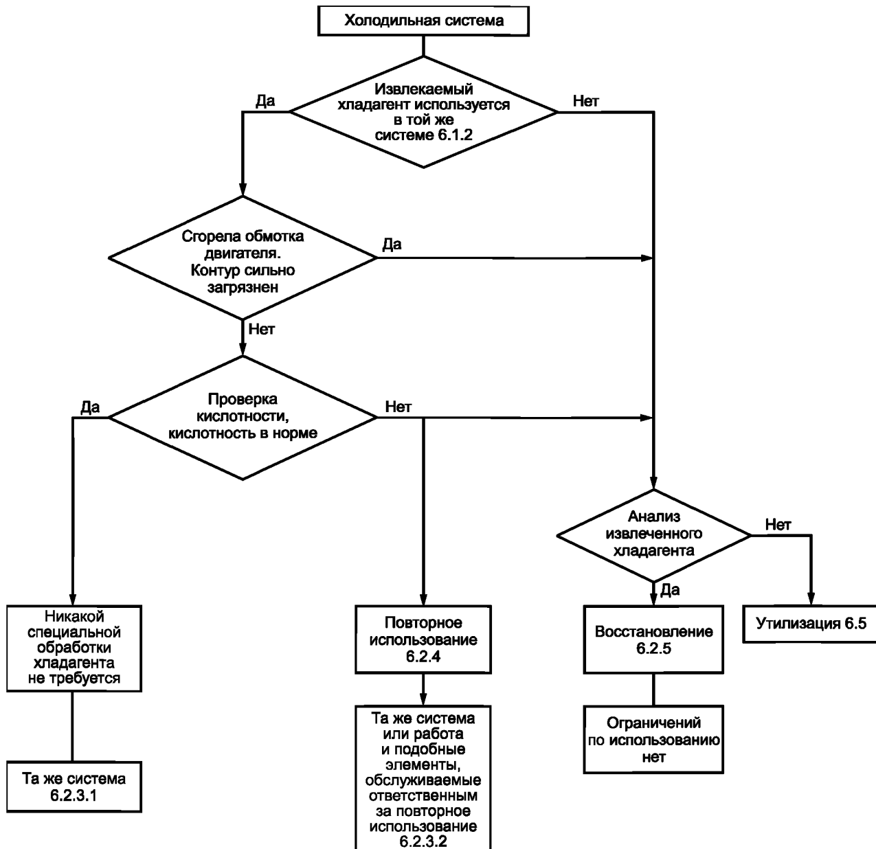
Рисунок 2 — Блок-схема операций, выполняемых при извлечении хладагента
