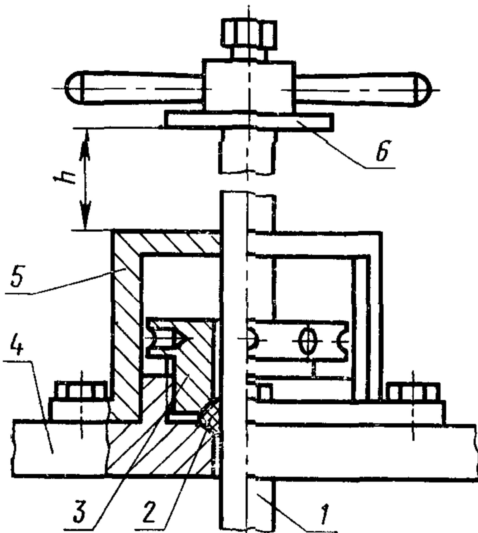
1 — штанга; 2 — набивка сальника, 3 — гайка, 4 — фланец; 5 — скоба; 6 — втулка
