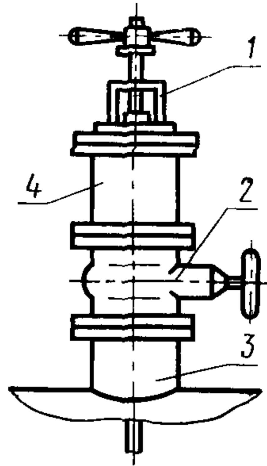
1 — сальниковый ввод; 2 — задвижка (затвор); 3 — патрубок; 4 — шлюзовая камера
